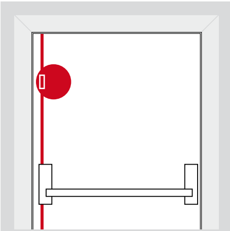
Montaż dla blokujących listew pionowych
